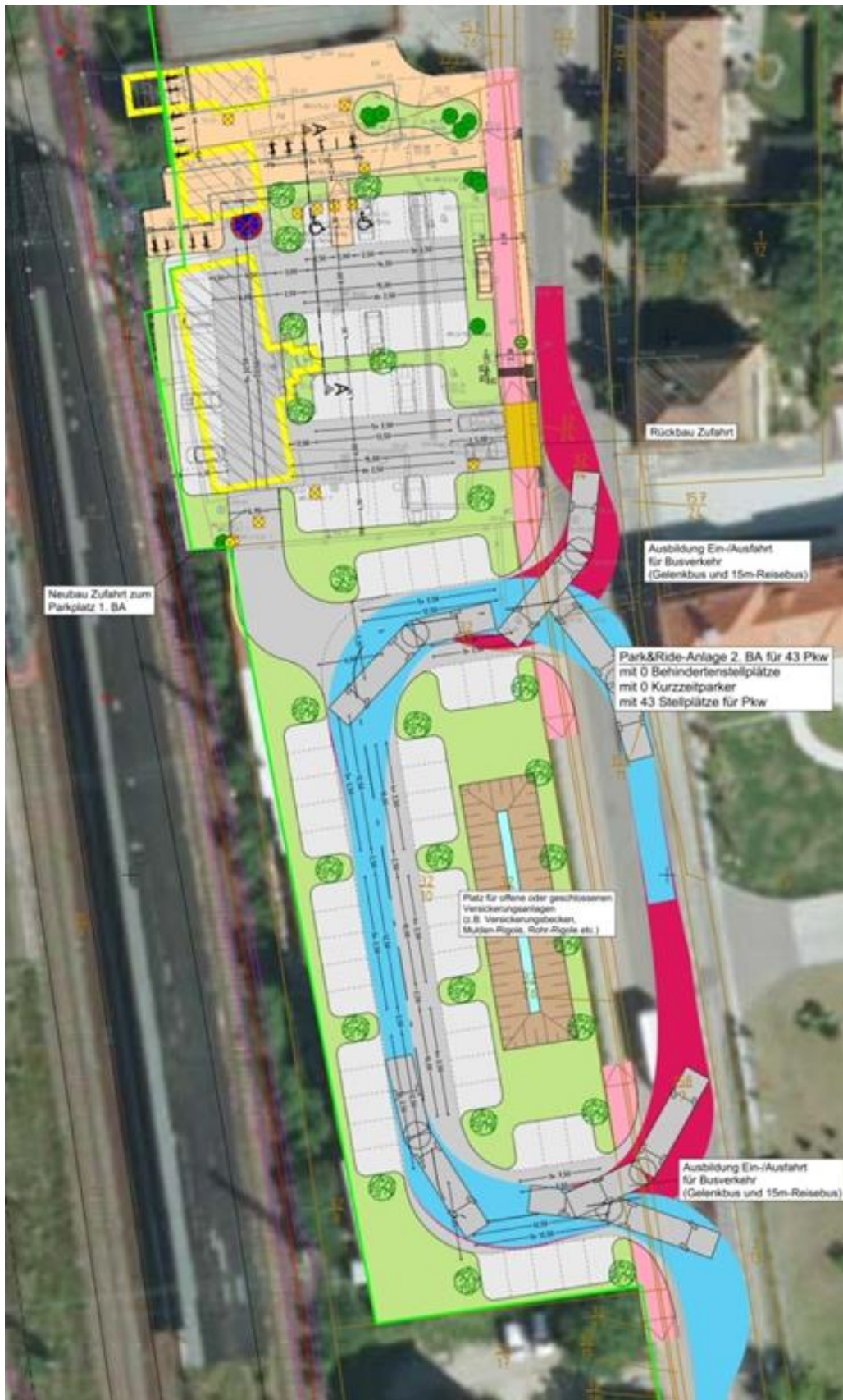
Abb.3: mögliche Gestaltung des ÖPNV-Verknüpfungspunktes mit Vorplatz, Buswendeschleife, und Stellplätze für Fahrräder und PKW (Quelle: xxxxxx)
