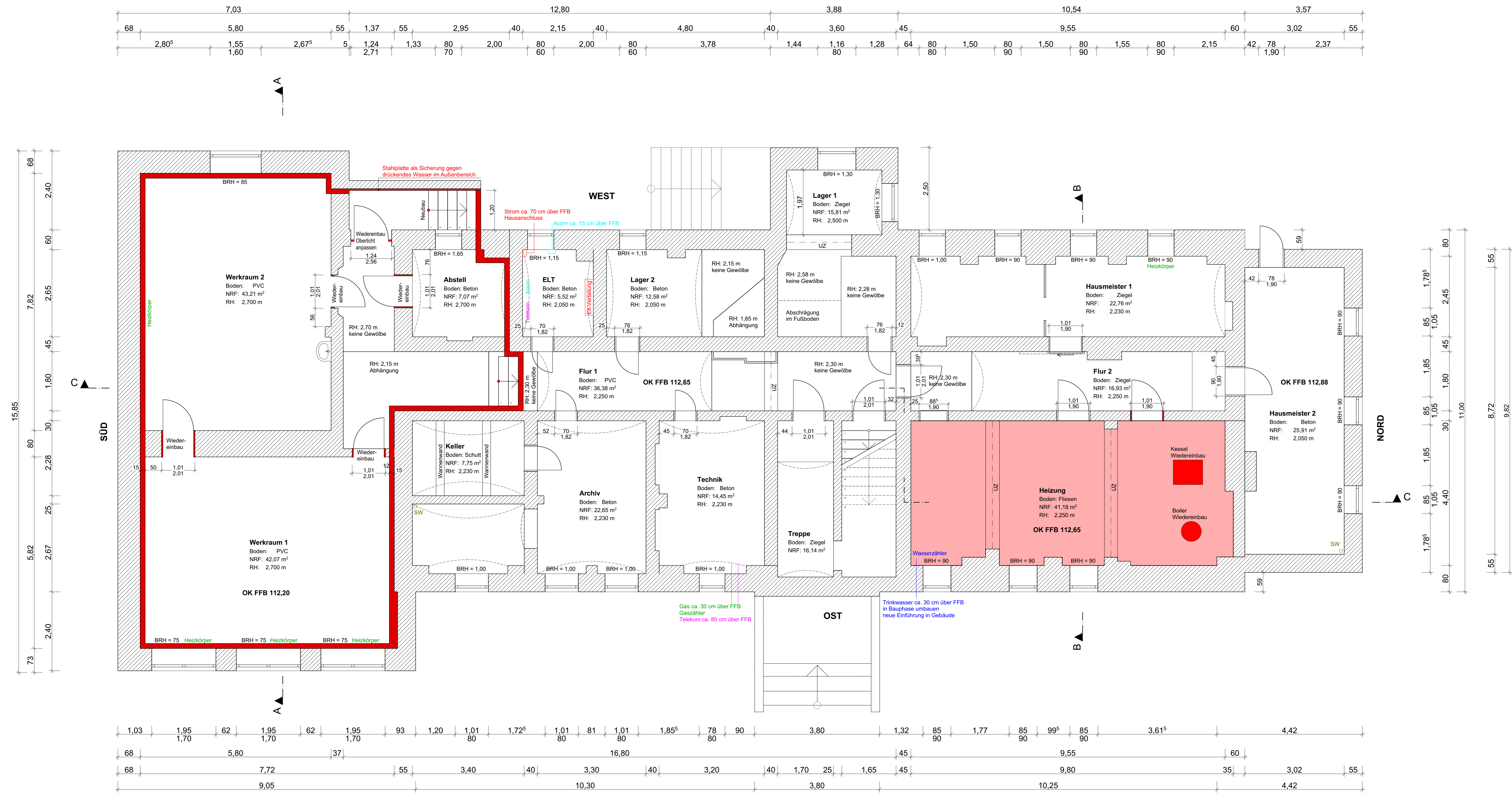
Kellergeschoss - innenliegende Schwarze Wanne in den Werkräumen und Teilverfüllung Heizungsraum Markkleeberg, Raschwitzer Straße 42 - Grundschule
