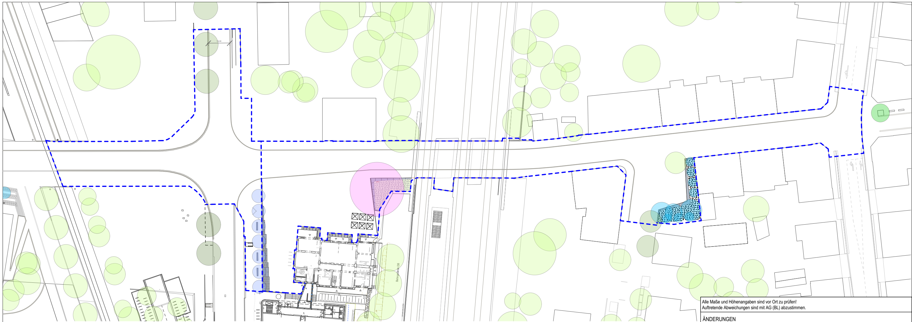
Lageplan Grenz- und Flächenabsteckung M1:750
